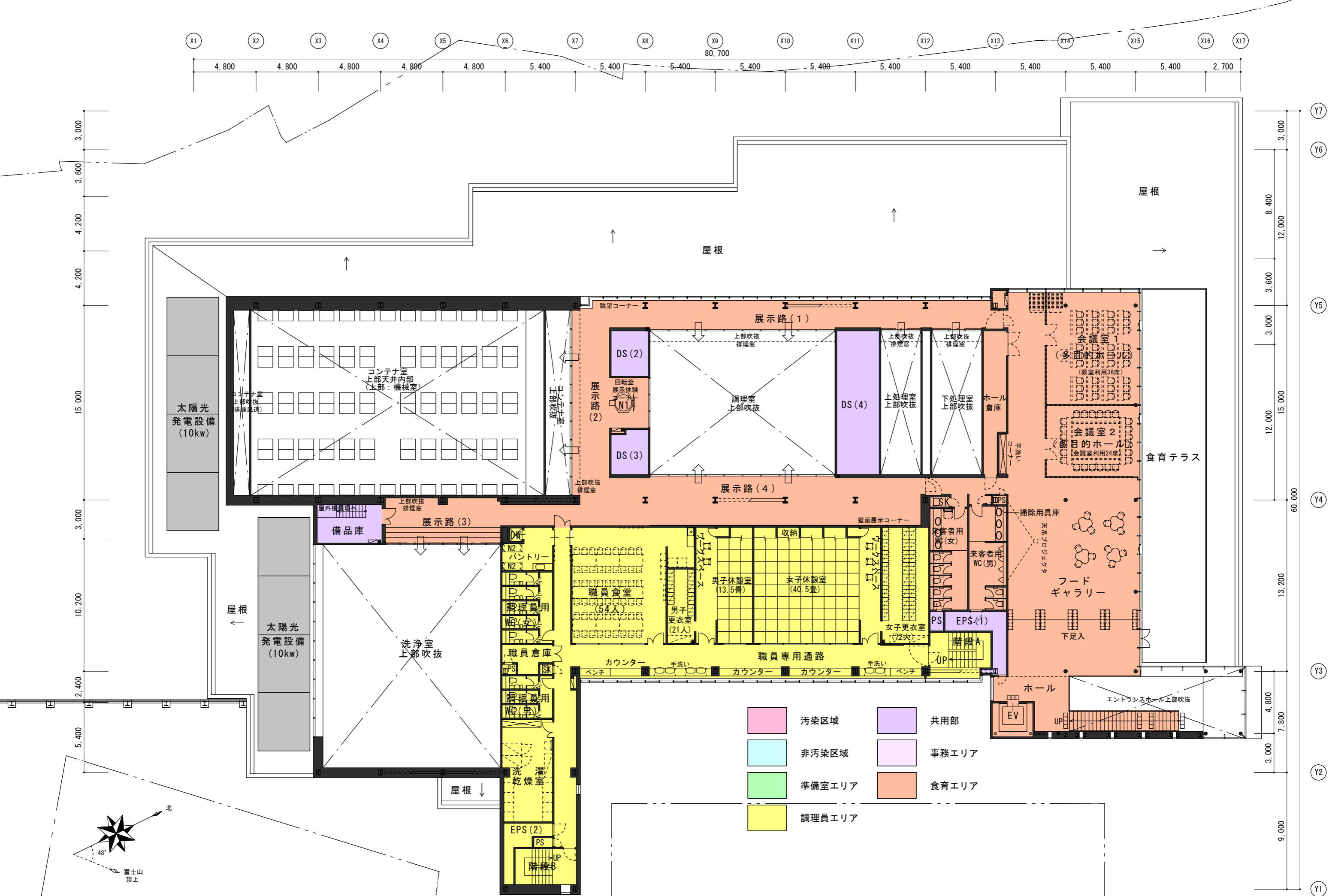
富士宮市立学校給食センター 2階平面図 S=1/250 (A3)
