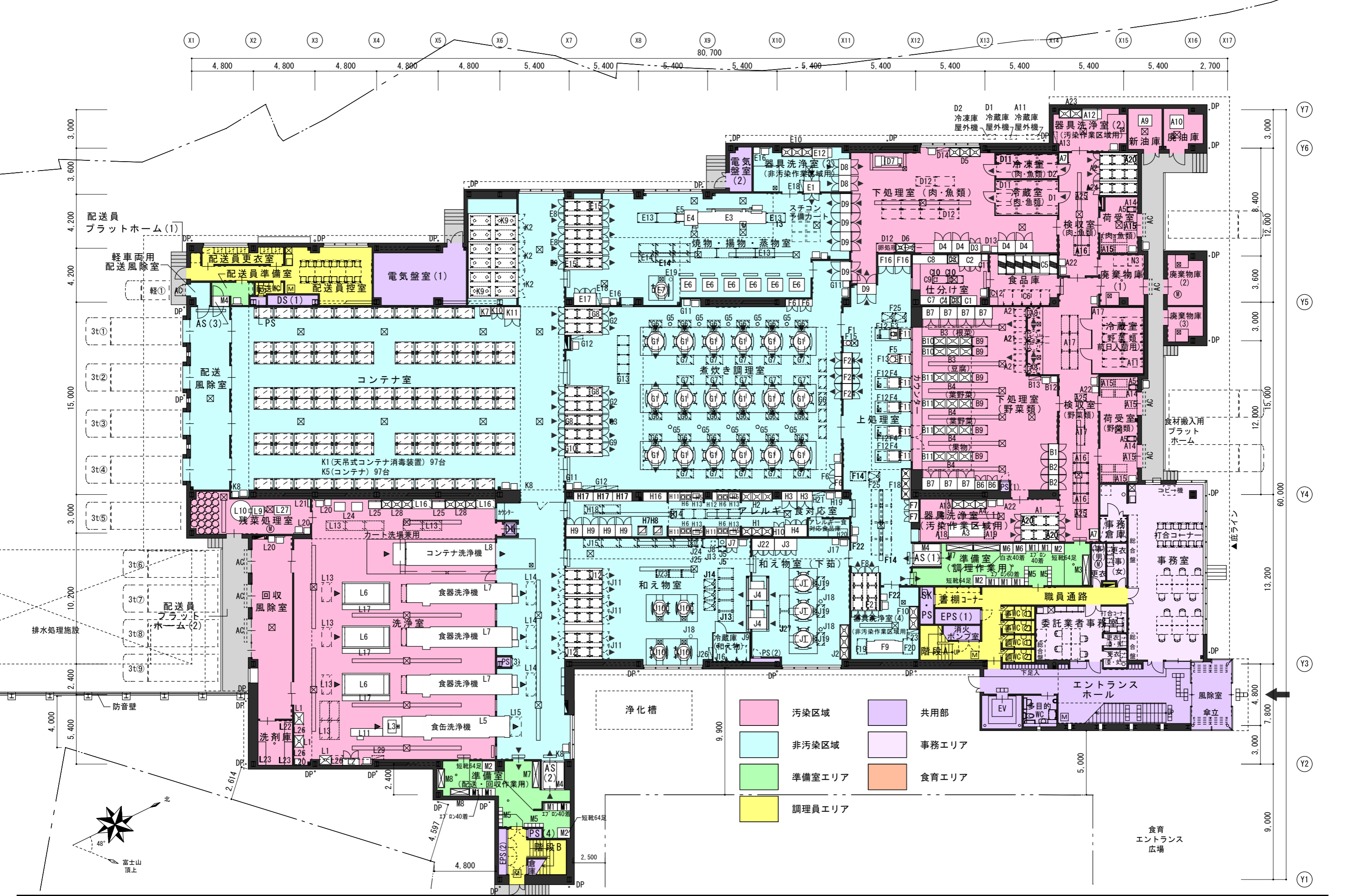
富士宮市立学校給食センター 1階平面図 S=1/250 (A3)
