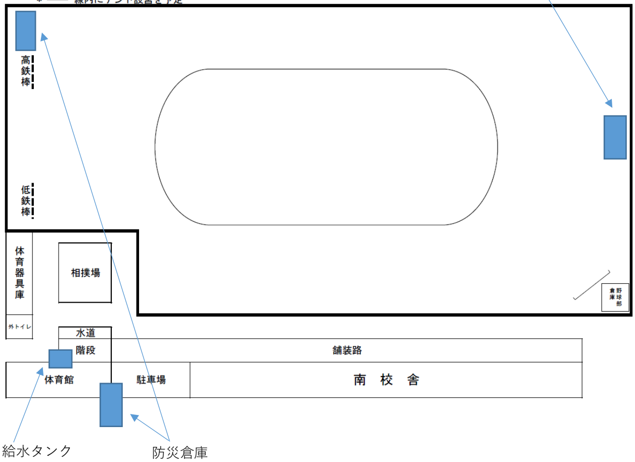
避難所開設時の学校開放区域図（グラウンド） * 線内にテント設置を予定
