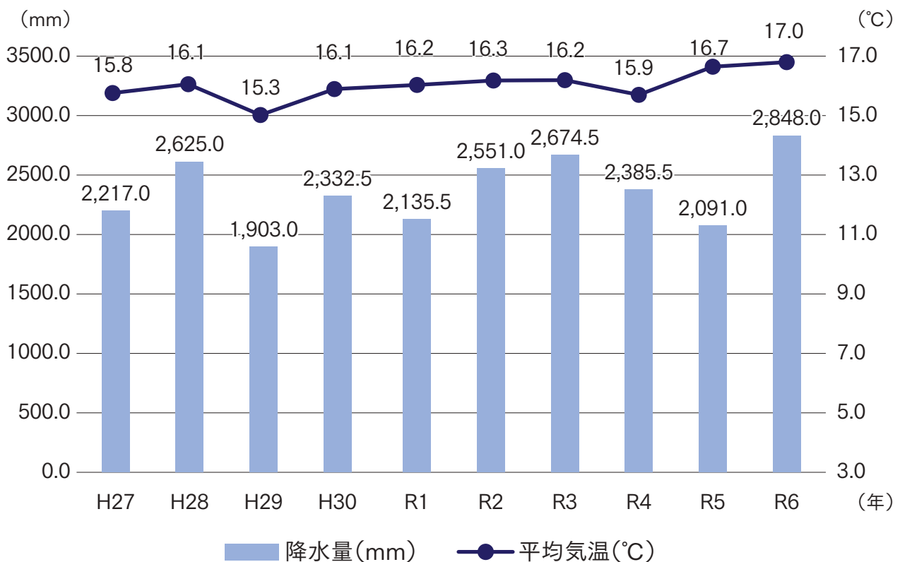
富士宮市の気候変化
