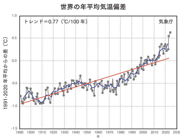
世界の平均気温の経年変化
