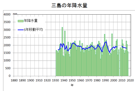
年降水量(三島)の経年変化
