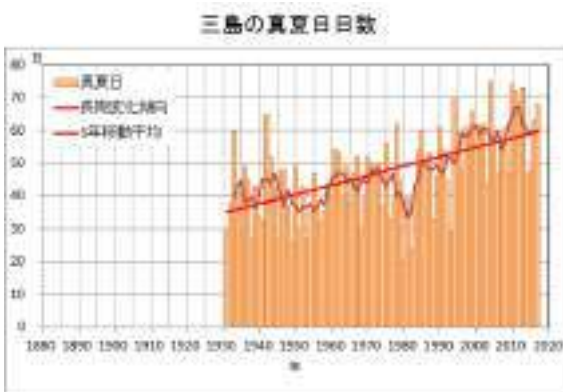
年間真夏日日数(三島)の経年変化
