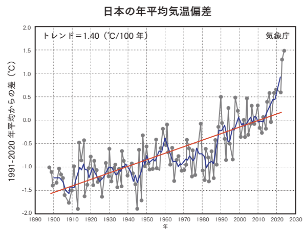
日本の平均気温の経年変化
