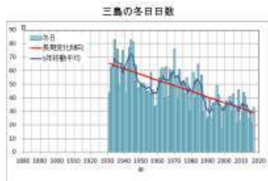
年間冬日日数(三島)の経年変化
