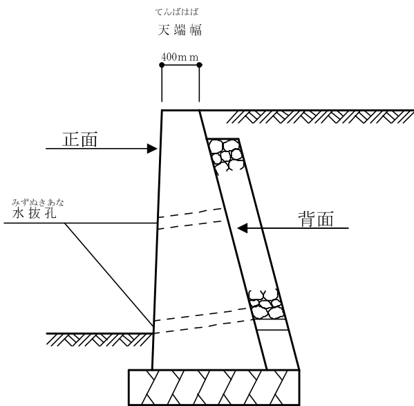
重力式コンクリート擁壁の例
