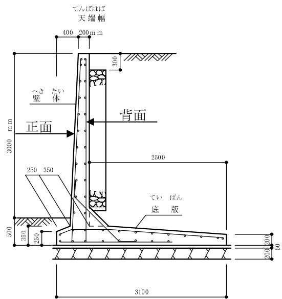
鉄筋コンクリートL型擁壁の例
